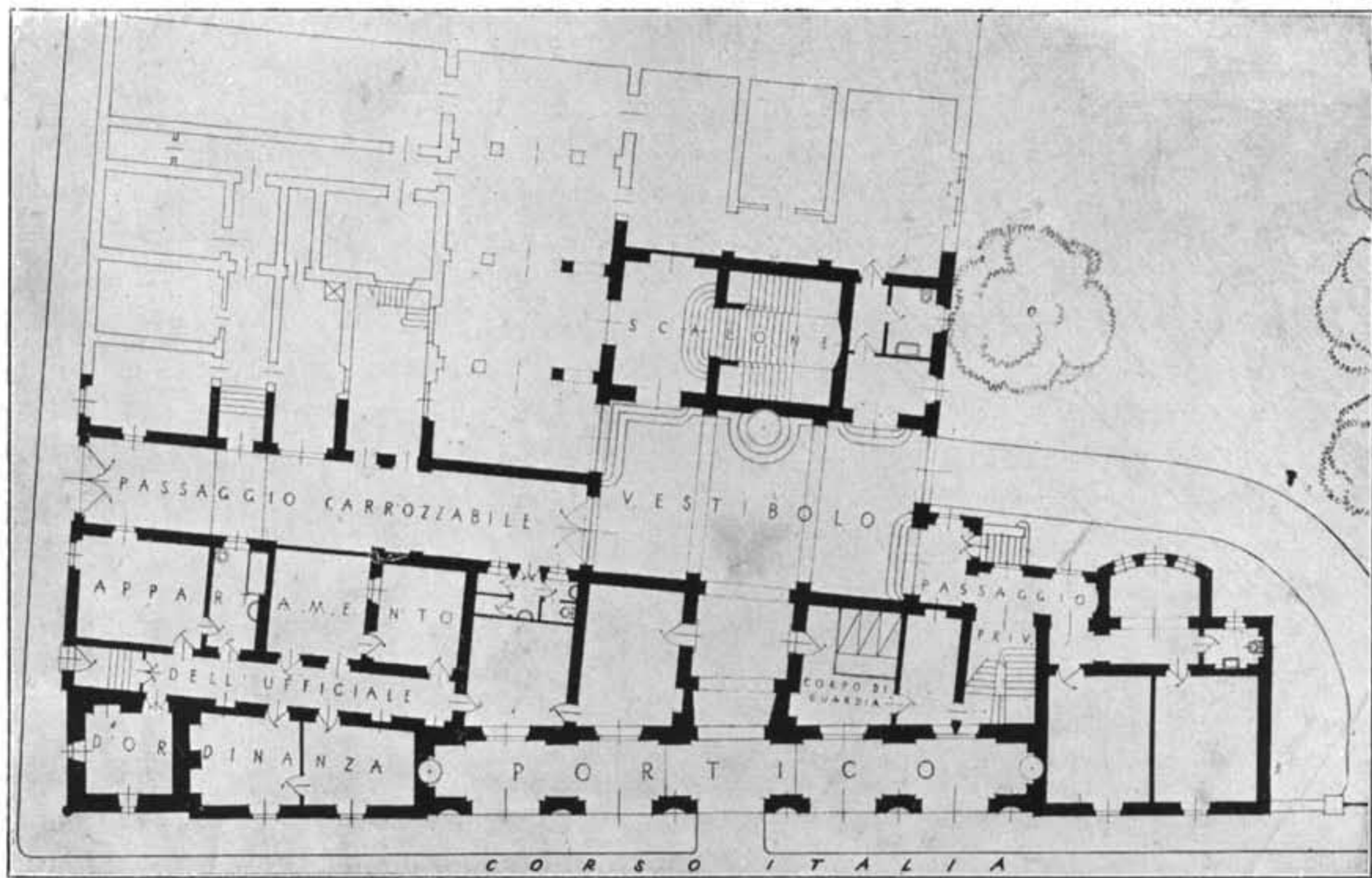
PROSPETTO (SOPRA). - PIANTA DEL PIANTERRENO (SOTTO).
